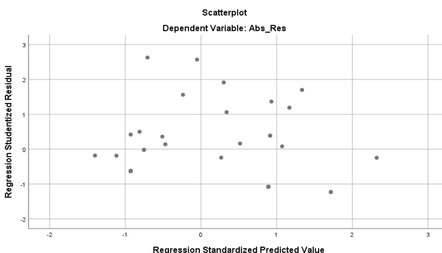
Gambar 1. Uji Heteroskedastisitas.
