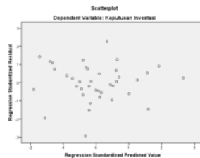
Gambar 1 Uji Heterokedastisitas
